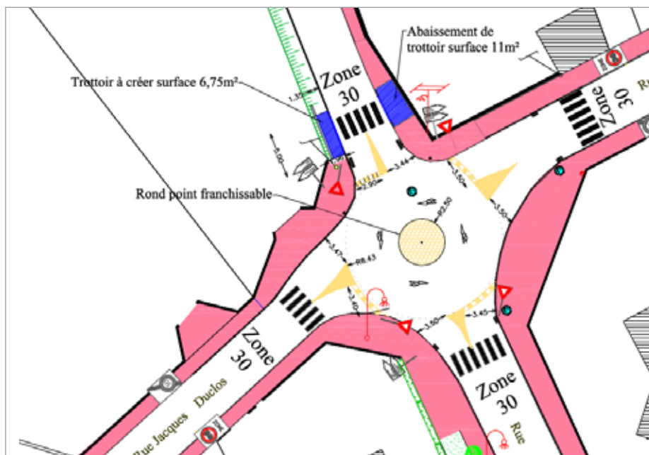
Schéma des futurs aménagements du carrefour de la rue Jacques Duclos et François Rabelais
